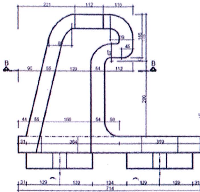
35 TONLUK BABA DETAYI
